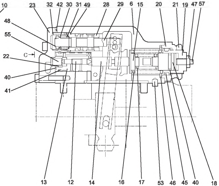
A-A KESİTİ SECTION A-A
