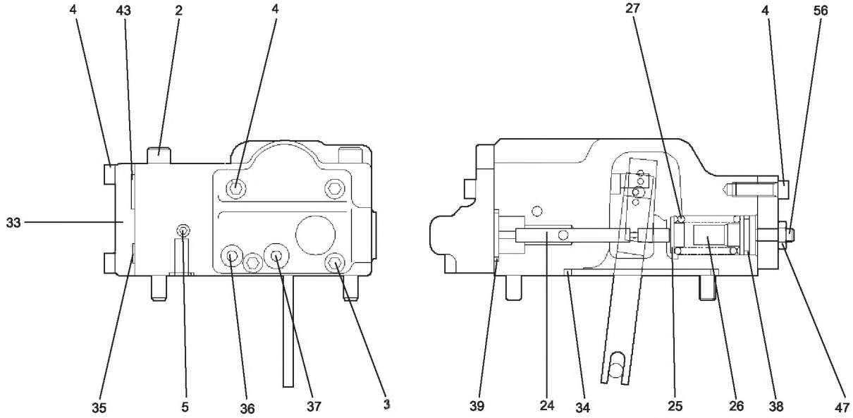
B-B KESİTİ SECTION B-B
